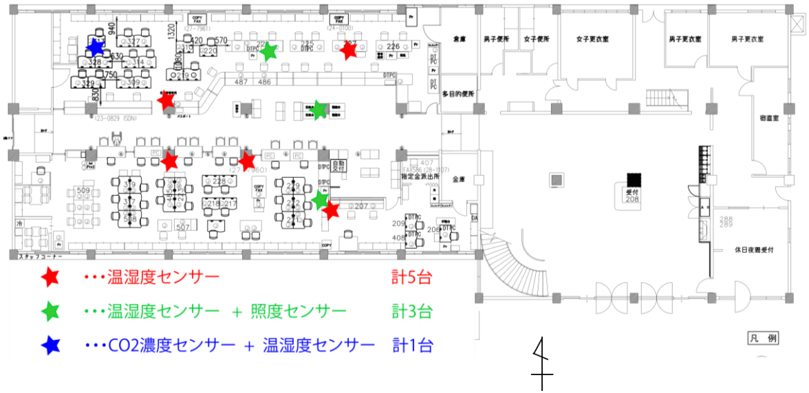
図 1.2.1 本館 1 階測定点
