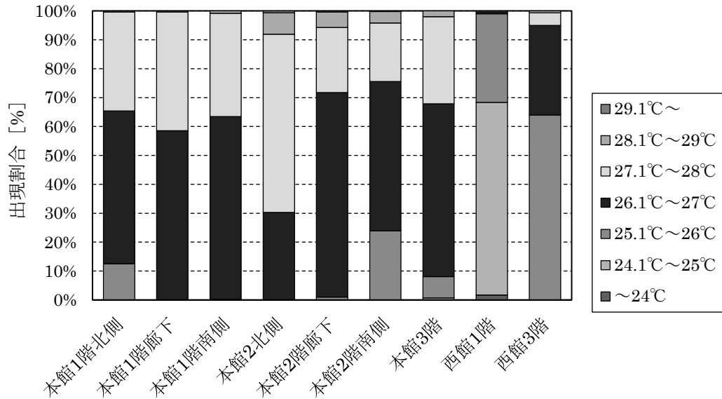
図 2.2.5 室内温度の出現割合
