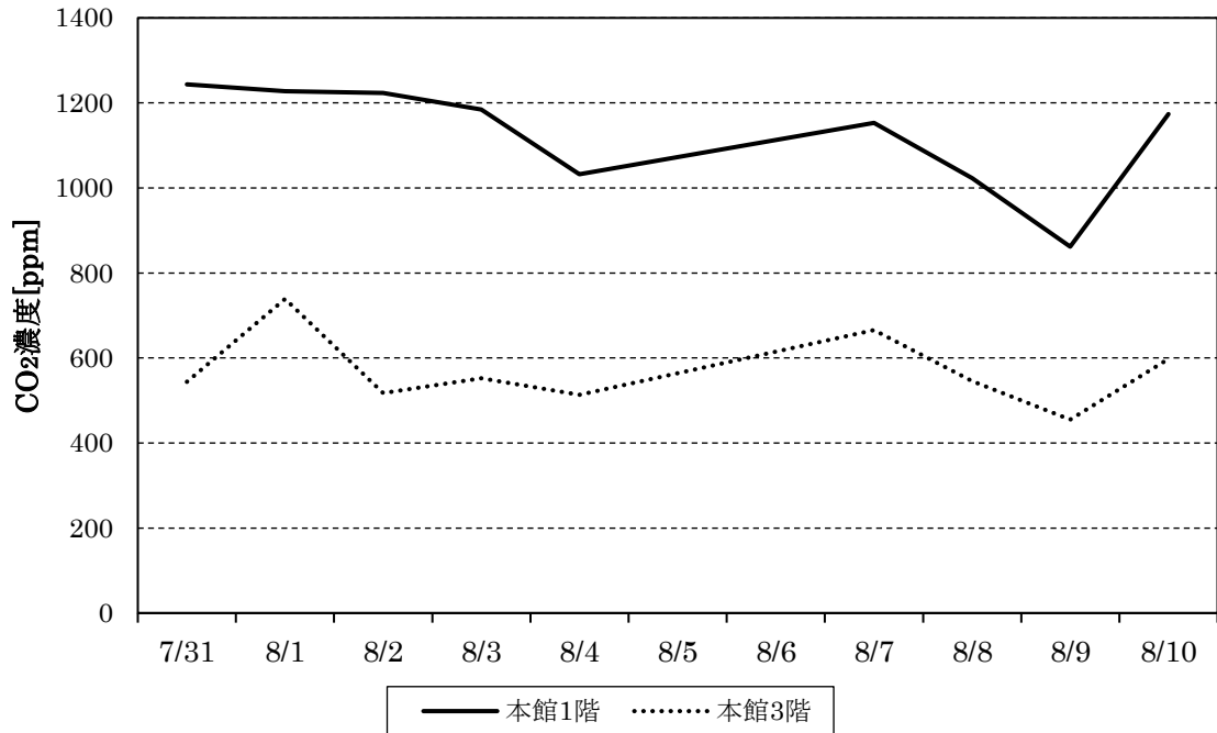
図 2.2.3 CO 2 濃度の測定結果
