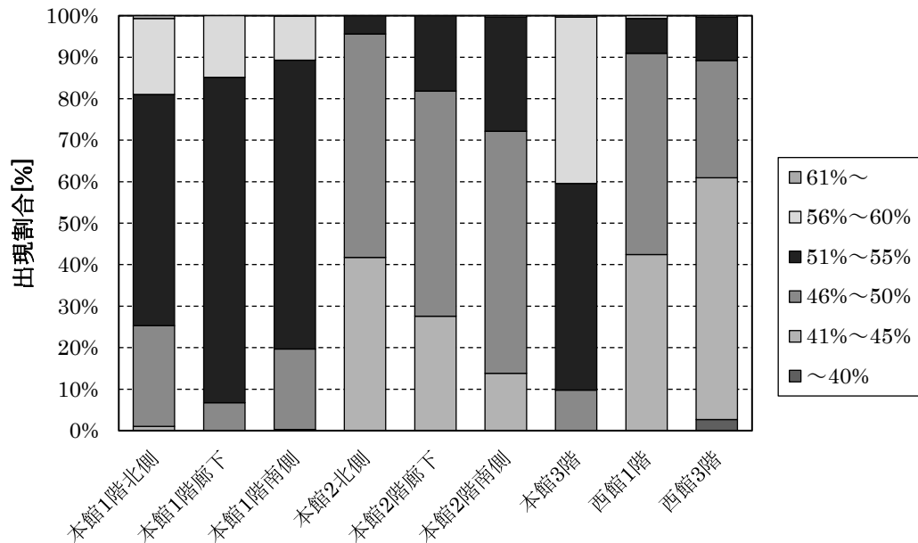
図 2.2.6 室内湿度の出現割合
