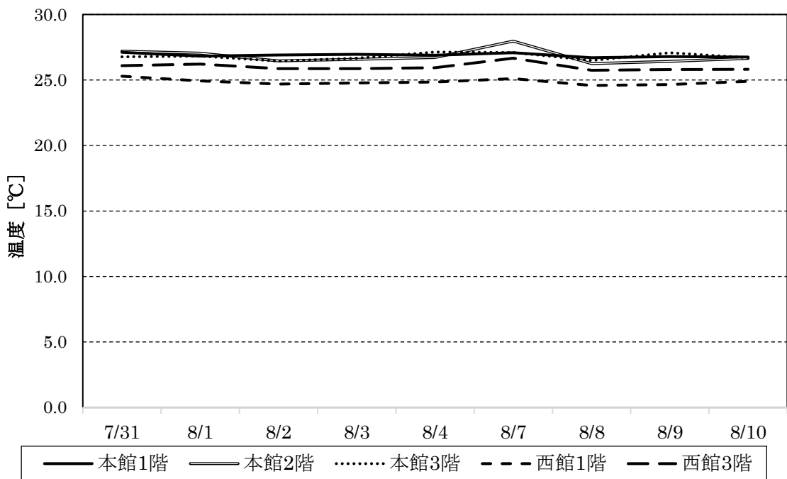
図 2.2.1 室内温度の測定結果
