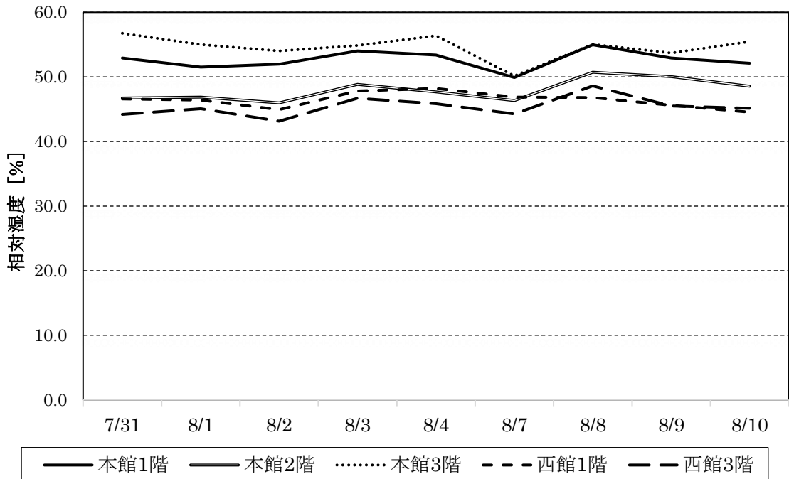
図 2.2.2 室内湿度の測定結果
