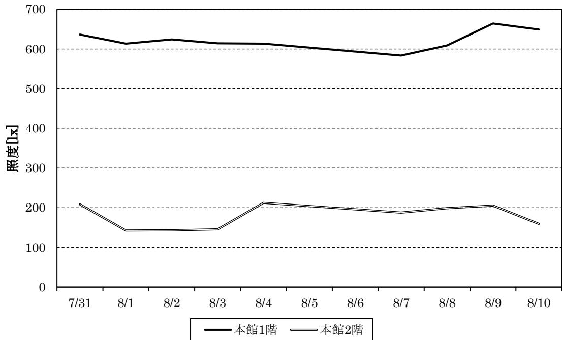
図 2.2.4 室内照度の測定結果
